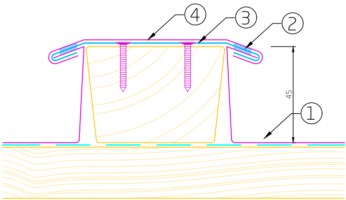
Deutsche Leistendeckung: ab 7° Dachneigung (lt. Deutscher Klempnerfachregeln) (Zusatzmaßnahmen empfohlen, siehe "Technische Informationen")
