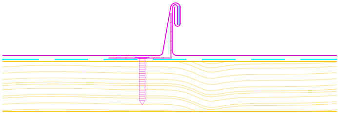
Doppelstehfalz: ab 7° Dachneigung (Zusatzmaßnahmen empfohlen, siehe "Technische Informationen")
