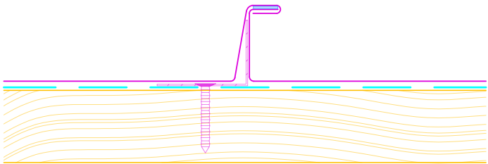
Winkelfalz: Mit Unterdach ab 25° Dachneigung. (Zusatzmaßnahmen empfohlen, siehe "Technische Informationen")
