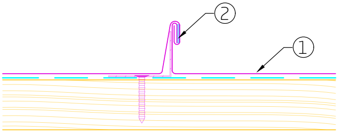
Doppelstehfalz: 3° - 7° Dachneigung mit Falzdichtmaßnahme
