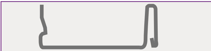
Schnappfalz 40 mm abgeflacht
