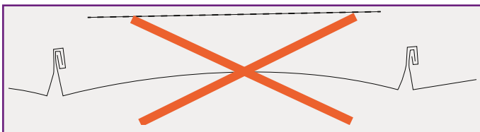
Aufwölbung der Scharen bei zu flachem Aufstellwinkel.
